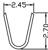
A-A SEC
